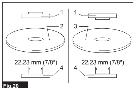
► 1. Contre-écrou 2. Meule tronçonneuse abrasive (plus mince que 4 mm (5/32")) 3. Meule tronçonneuse abrasive (4 mm (5/32") ou plus épaisse)
