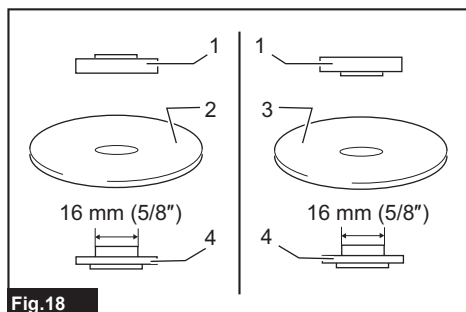
► 1. Contre-écrou 2. Meule tronçonneuse abrasive (plus mince que 4 mm (5/32")) 3. Meule tronçonneuse abrasive (4 mm (5/32") ou plus épaisse) 4. Flasque intérieur
